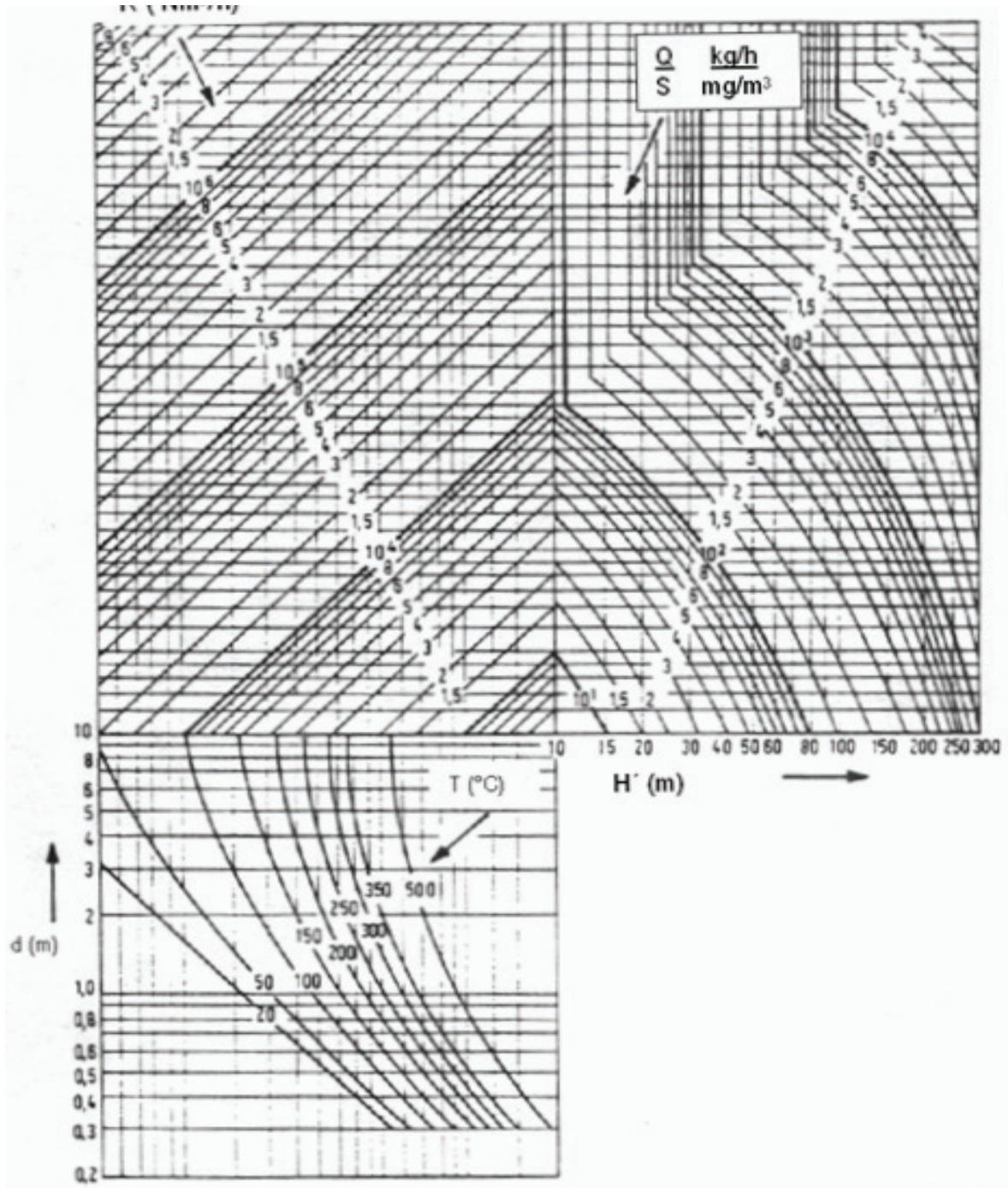
Gráfica 1. Nomograma para el cálculo de la altura mínima de chimenea.
